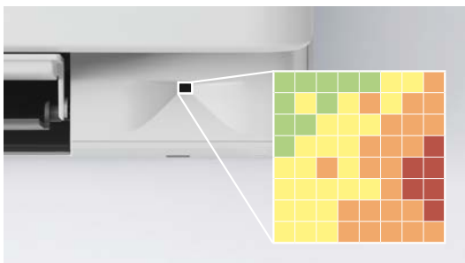
Der intelligente Thermo- und Bewegungssensor unterteilt die Raumbofläche in 64 Quadrate, um ihre Temperatur genau zu bestimmen.
